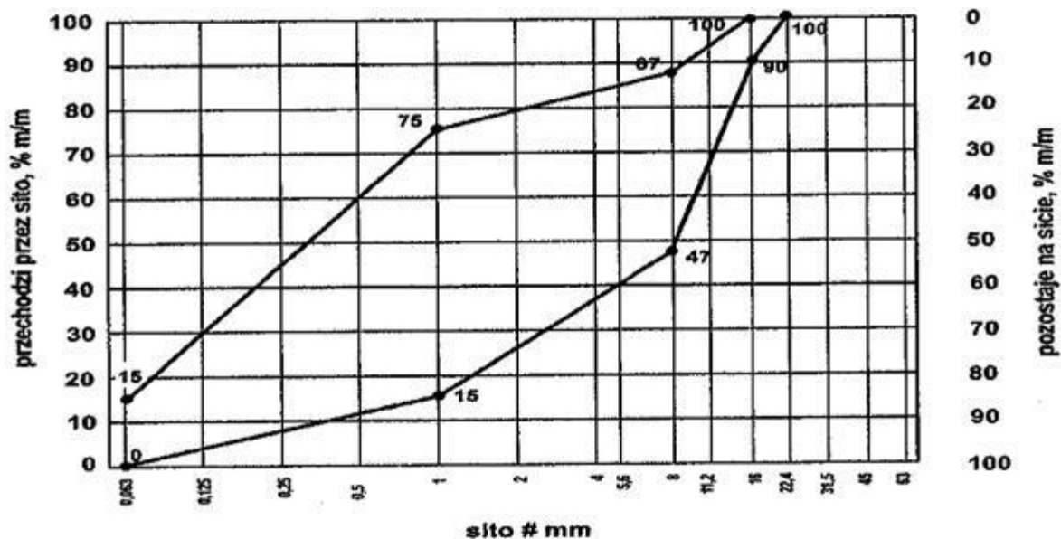
Rys. 3. Krzywe graniczne uziarnienia mieszanki kruszyw 0/16 mm do górnej warstwy podłoża ulepszzonego
